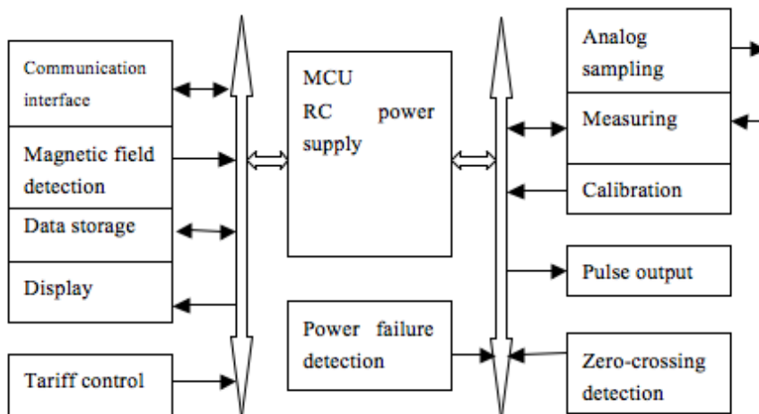
Bild 14: Blockdiagramm DxS74
