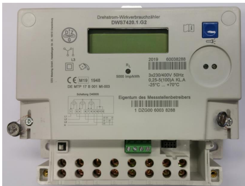
Bild 7: Gehäuseschrauben mit Plastik-kappen
