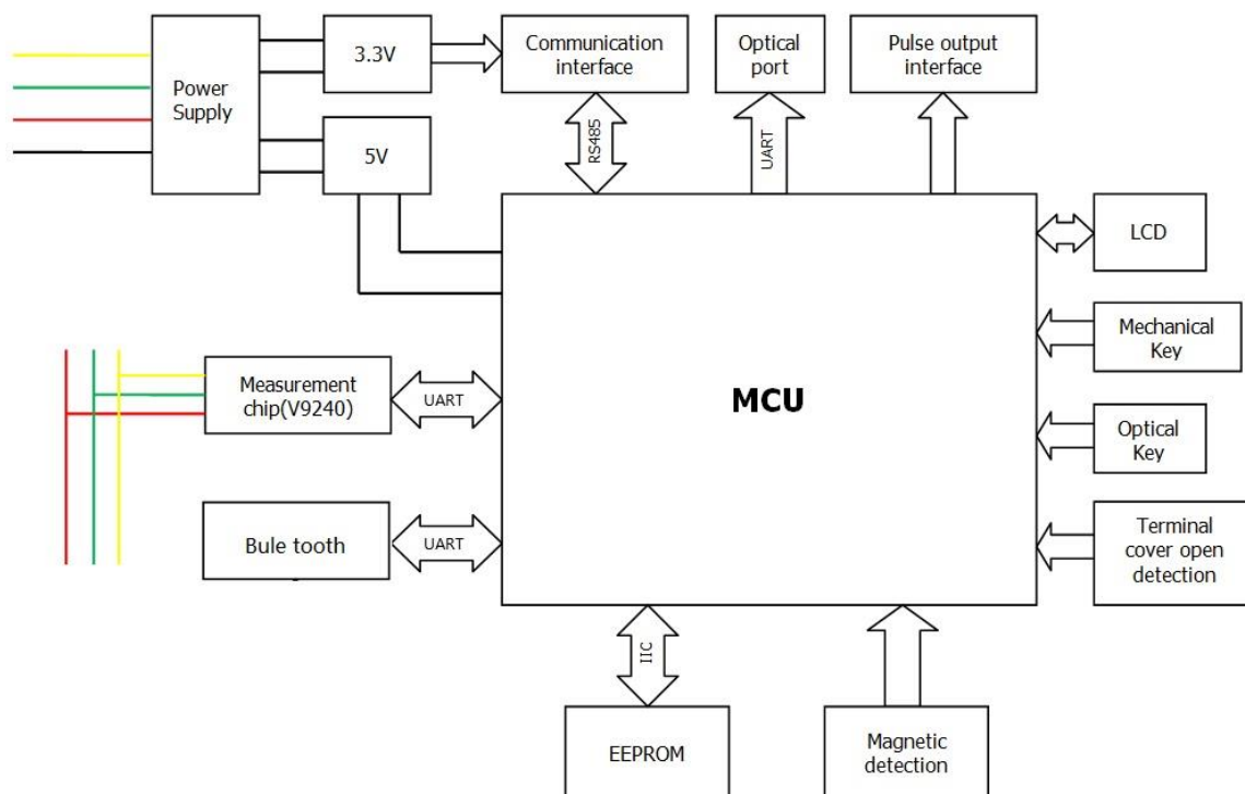
Bild 15: Blockdiagramm DxS74.G2
