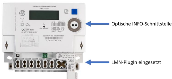
Bild 12: Schnittstellen (DVS74 mit LMN-Plugin)
