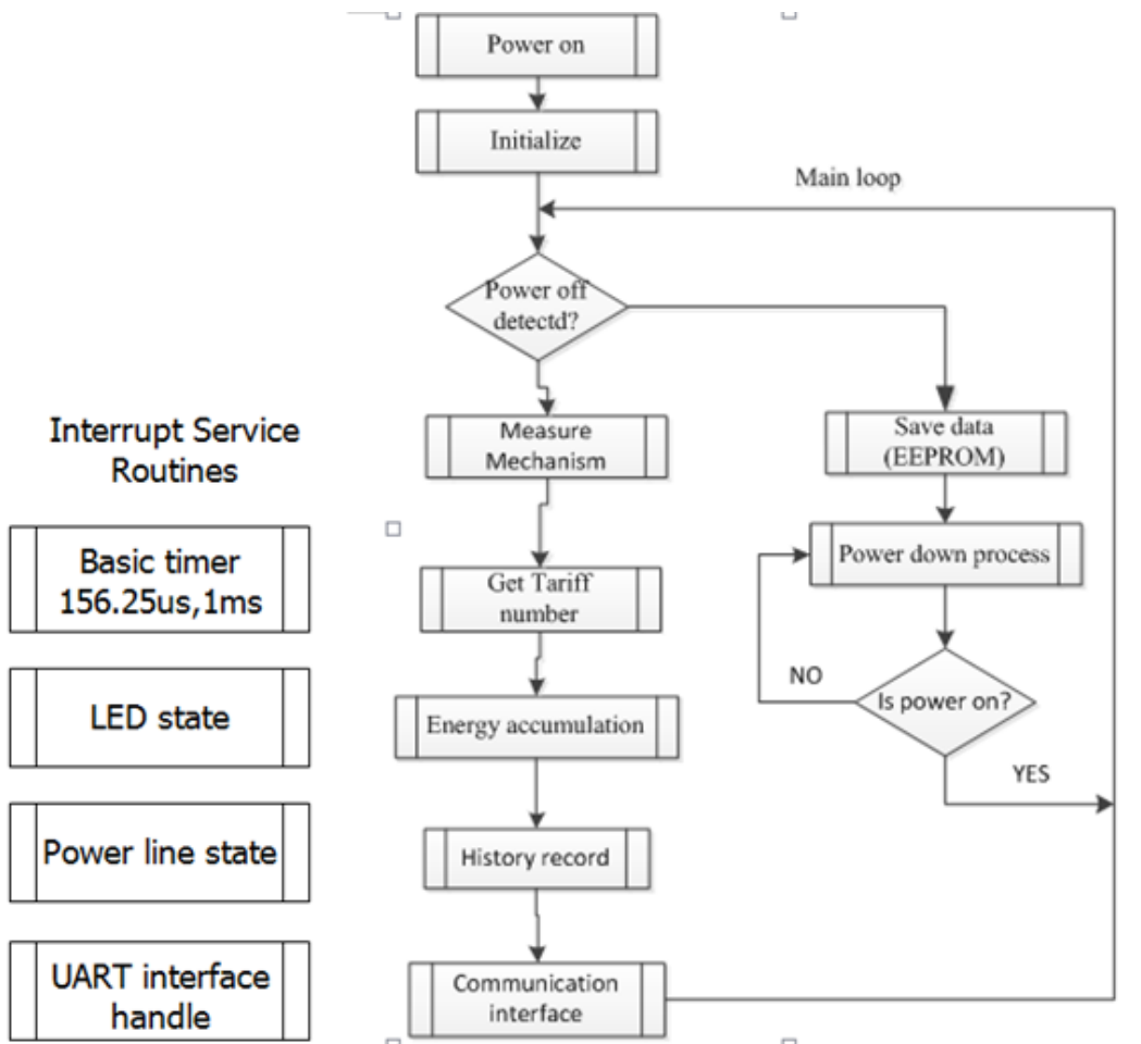
Bild 17: Firmware Flussbild
