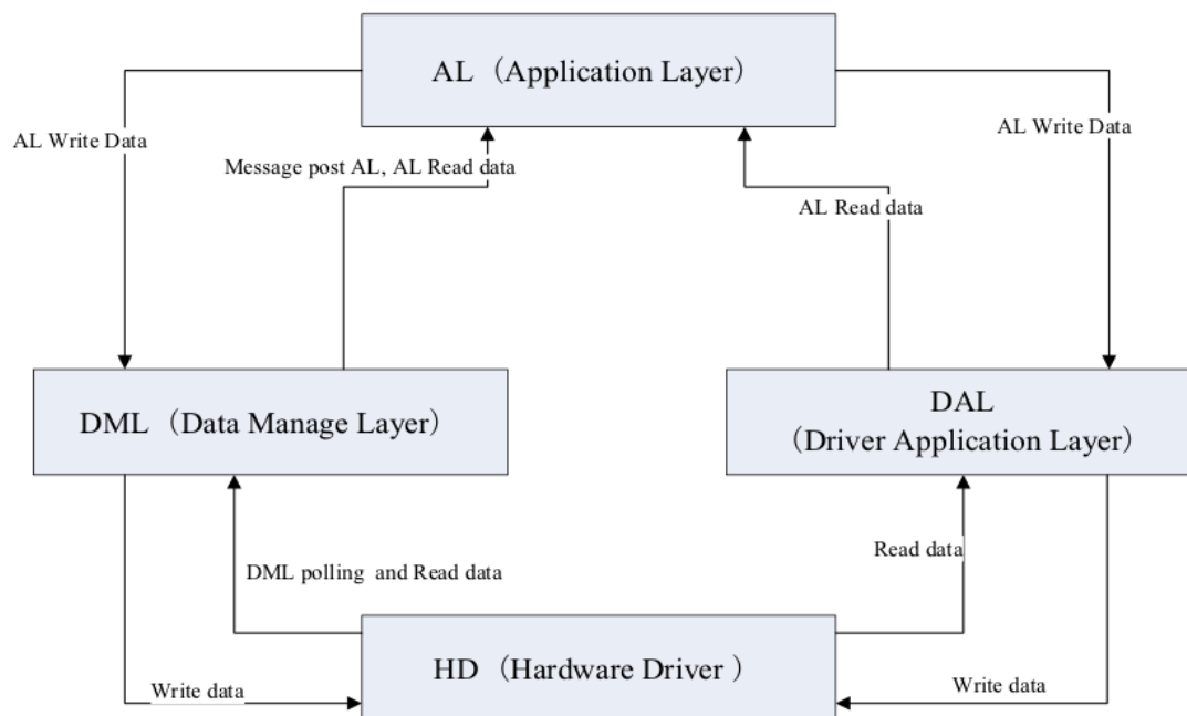
Bild 16: Struktur der Firmware
