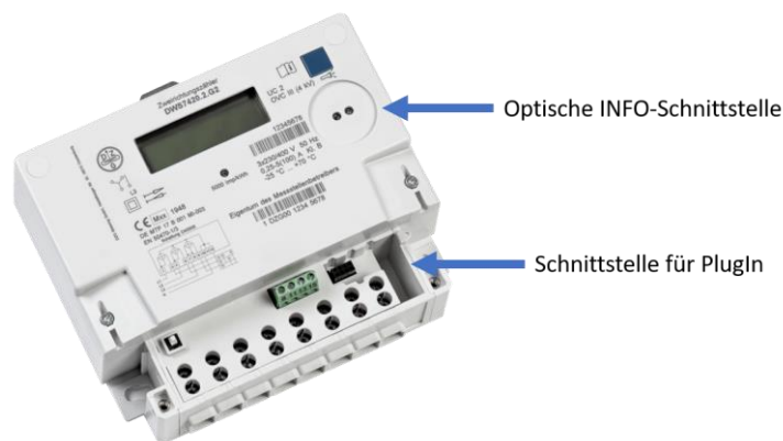
Bild 11: Optische und PlugIn-Schnittstelle (DWS74.G2)
