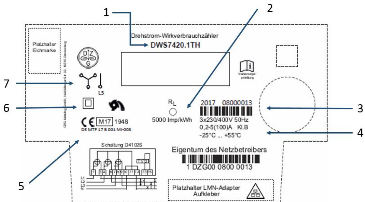
Bild 9: Leistungsschild
