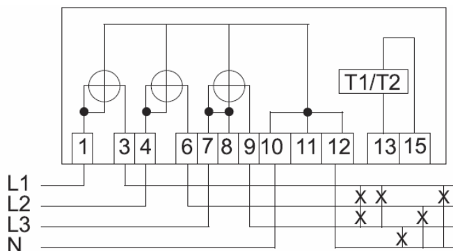
Bild 5: Schaltbild
