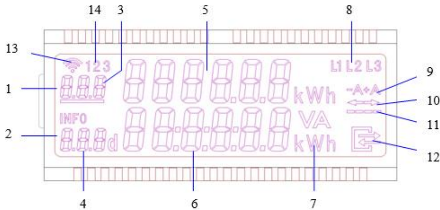
Fig. 8: LCD
