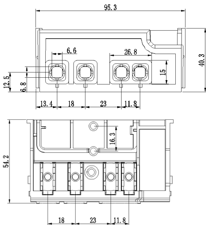
Fig. 3: Klemmenblock
