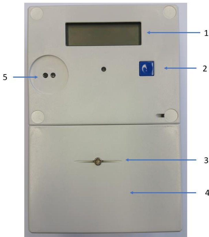
Fig. 1: Gehäuse
