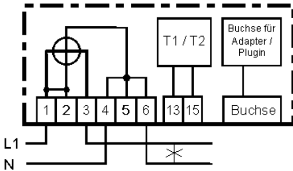
Fig. 4: Schaltbild
