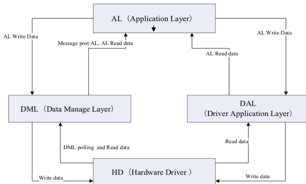
Fig. 10: Firmware Struktur
