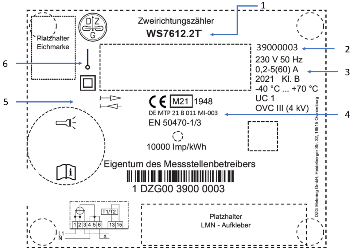
Fig. 7: Leistungsschild
