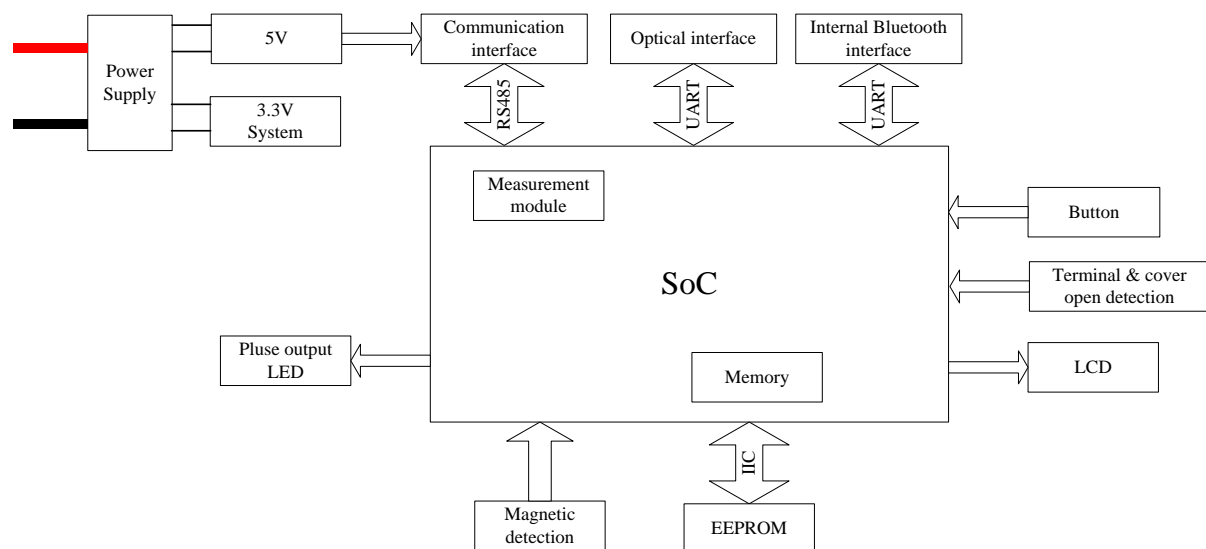
Fig. 9: Blockdiagramm
