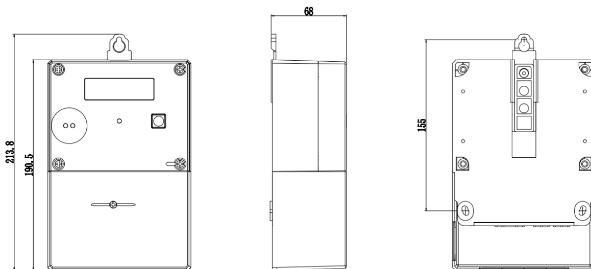
Fig. 2: Abmessungen Gehäuse
