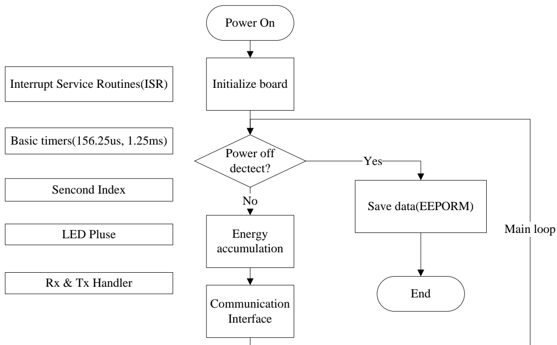
Fig. 11: Firmware Flussbild
